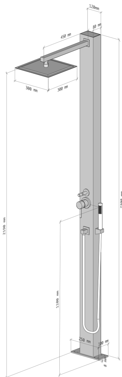
Technische Darstellung der Standardausführung · Masse in Millimetern
